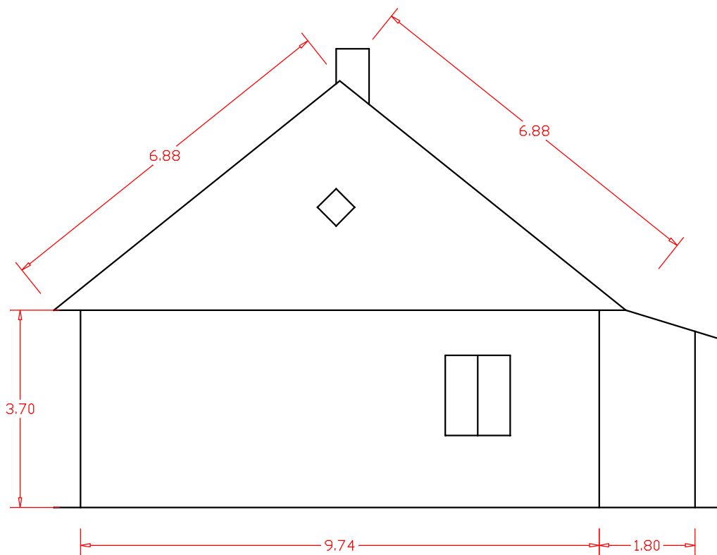
Szkola w Cygance, elewacja boczna, skala 1: 100
