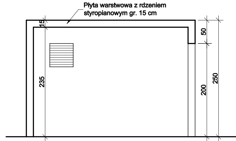
Przekrój A-A, 1:50
